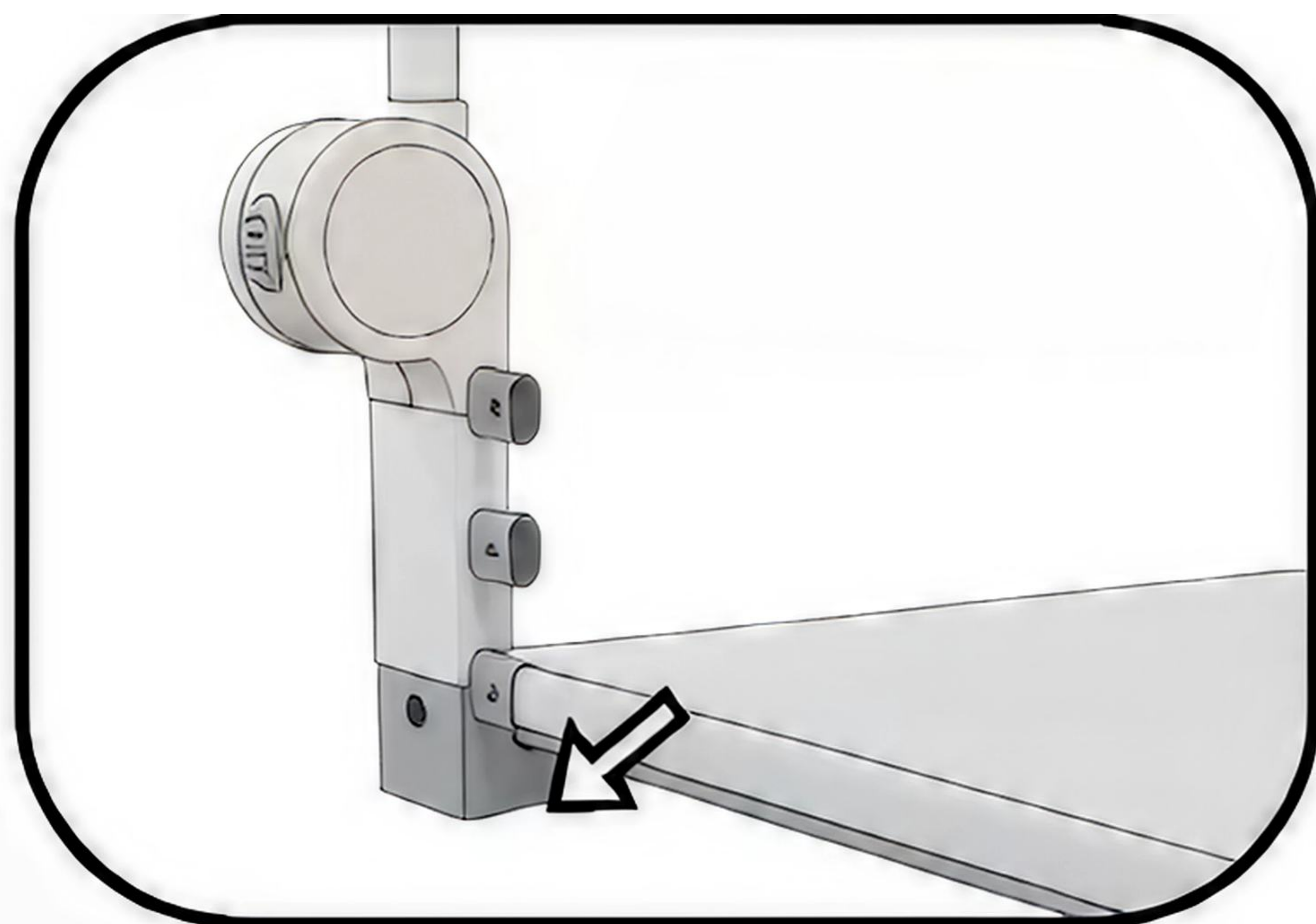
Установка поперечной трубы для тонкого матраса.
